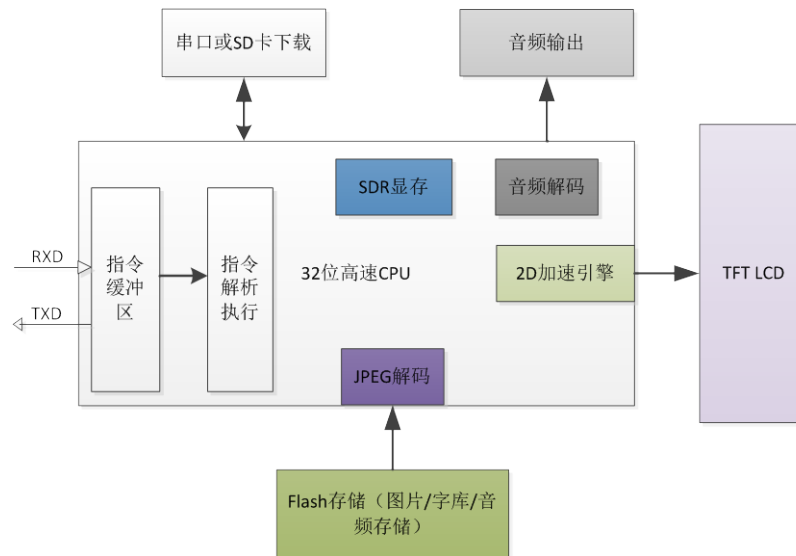
图 9-1 M 系列串口屏内部结构图
