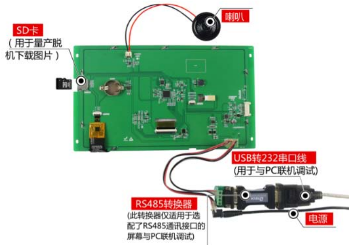
图 1-5 调试工具图
