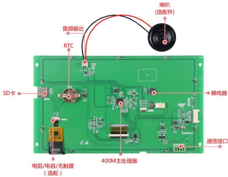
图 1-4 硬件配置图
